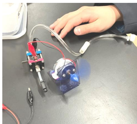
燃料電池キットでの発電実験
